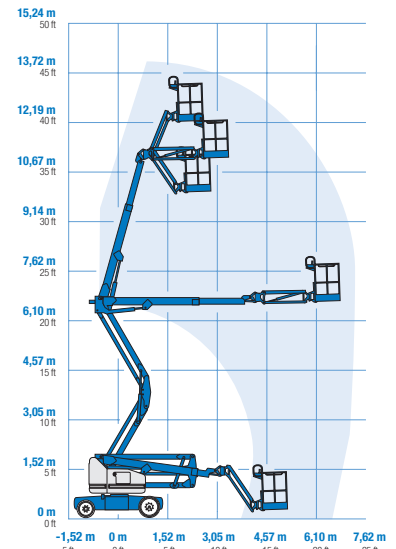
Arbeitsdiagramm Z-40/23N RJ
