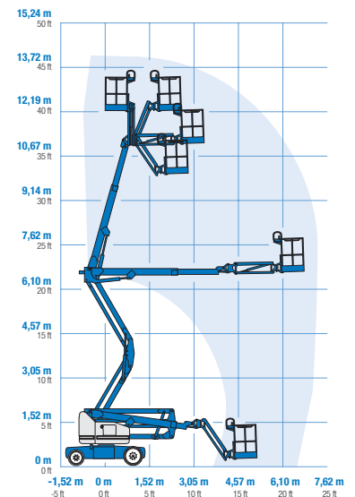
Arbeitsdiagramm des Korbarms Z-40/23N RJ
