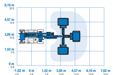
Arbeitsdiagramm des Korbarms Z-40/23N RJ
